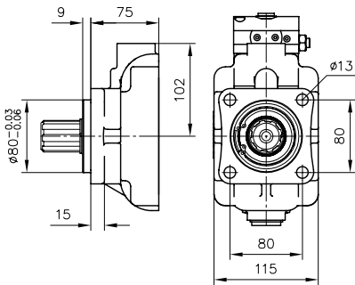
Coding Y (ISO 7653-1985)
