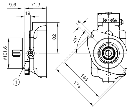
Coding X (SAE-B 2-hole) (101-2 ISO 3019-1)
